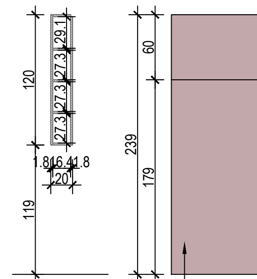
PRESJEK 1 - 1
