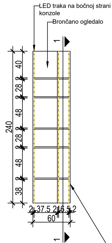
KONZOLA - POGLED
