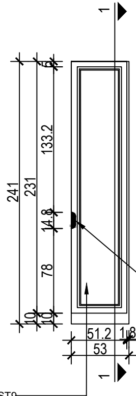
SKLADIŠNI ELEMENT - POGLED
