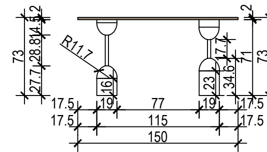
KONZOLNI STOL - POGLED
