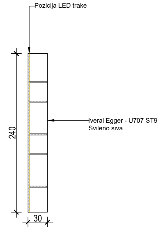
PRESJEK 1-1
