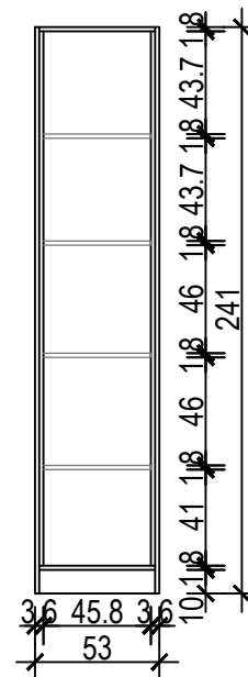
SKLADIŠNI ELEMENT - KORPUS
