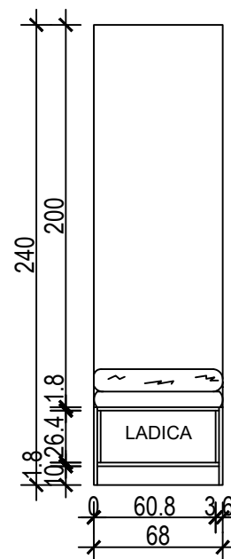
KLUPICA - KORPUS
