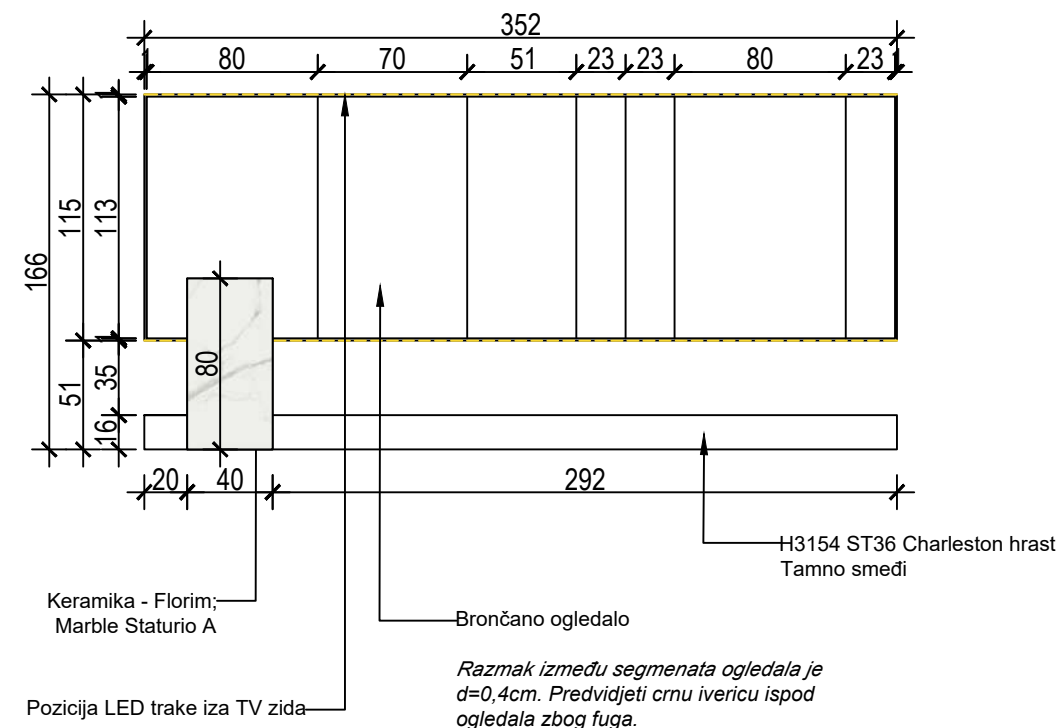
TV ZID I TV KLUPA - POGLED
