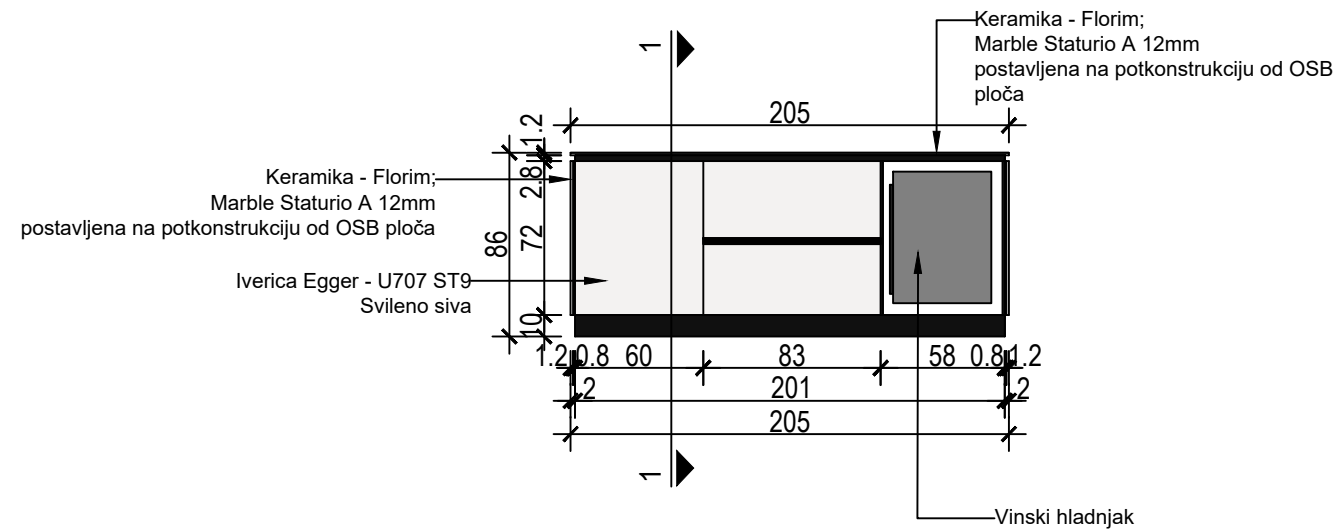
OTOK - POGLED
