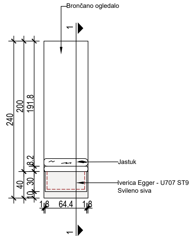
KLUPICA - KORPUS
