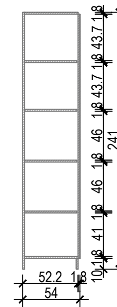
PRESJEK 1-1
