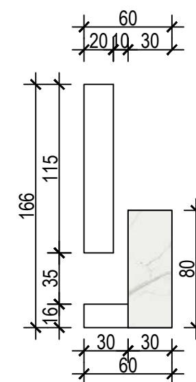
TV ZID I TV KLUPA - BOČNI POGLED
