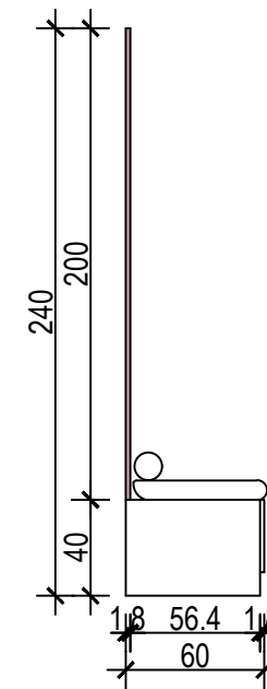
PRESJEK 1 - 1
