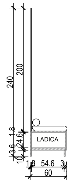
PRESJEK 1 - 1
