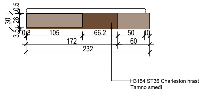
KLUPICA ZA SJEDENJE - POGLED
