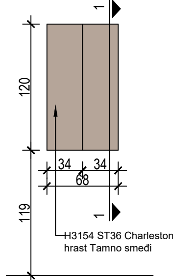
POGLED
