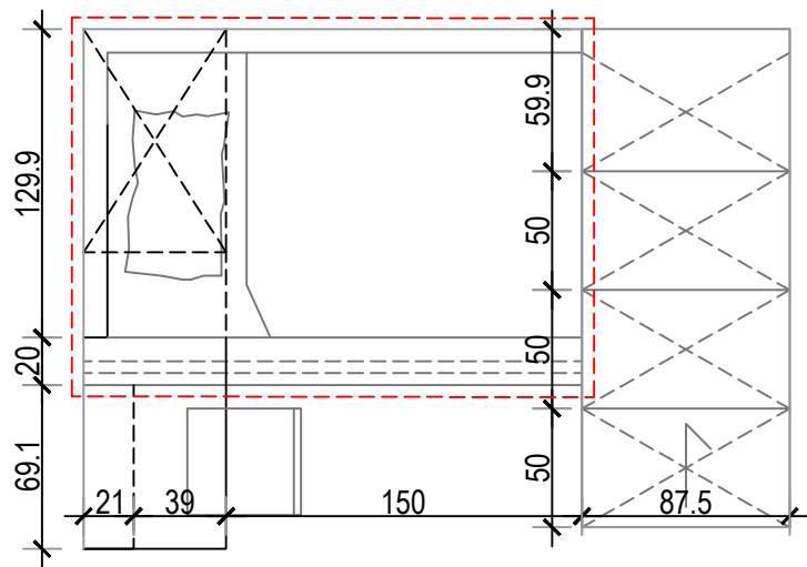
KREVET - TLOCRT
