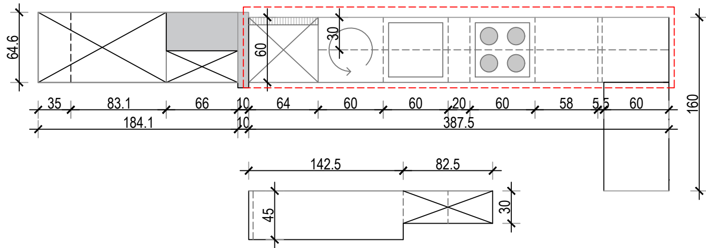
KUHINJA - TLOCRT
