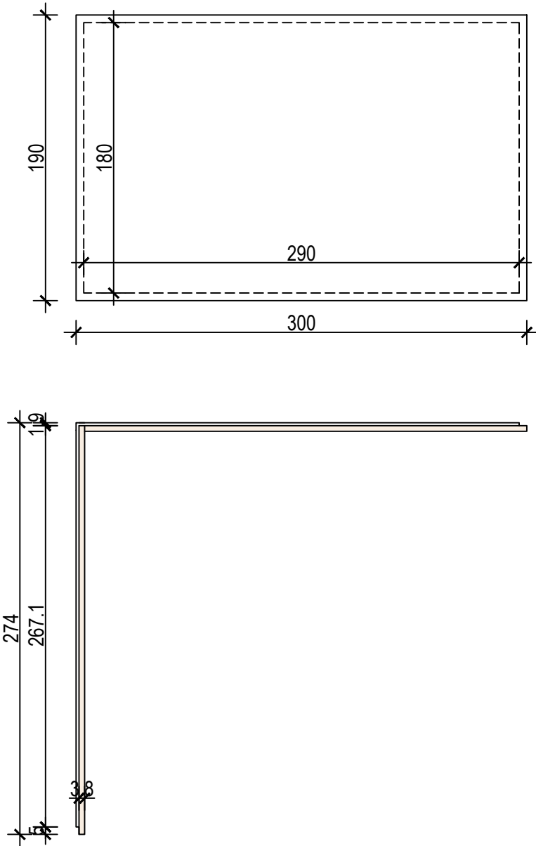
ELEMENT - TLOCRT
