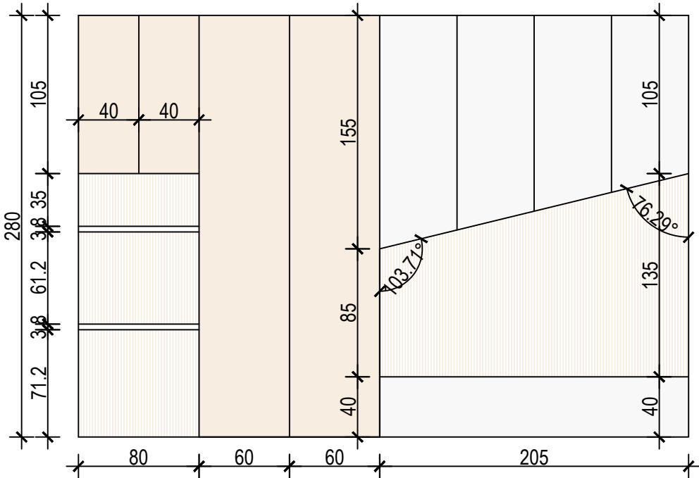
ORMAR - POGLED
