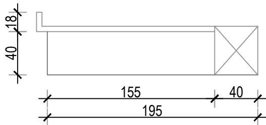
'TV WALL' - TLOCRT
