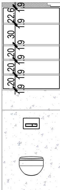
POGLED 1 - KORPUS
