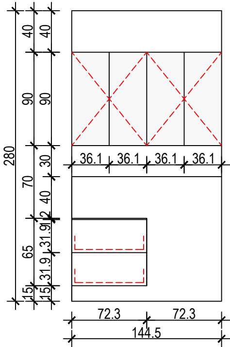
ORMAR - POGLED
