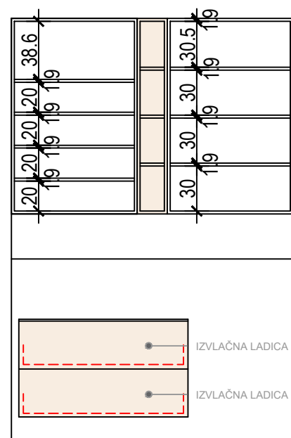
ELEMENT - KORPUS
