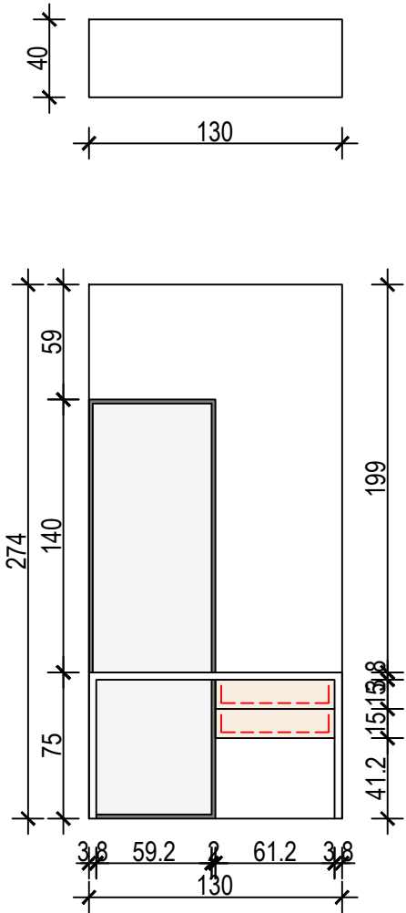
ELEMENT - TLOCRT
