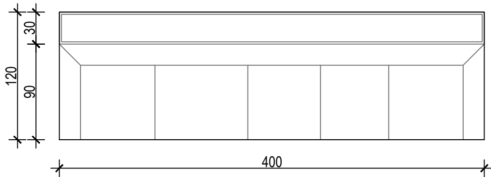
SEPRE - TLOCRT
