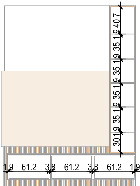
'TV WALL' - KORPUS
