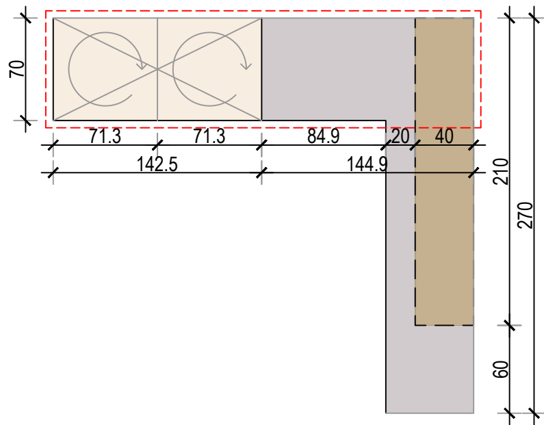
ELEMENT - TLOCRT
