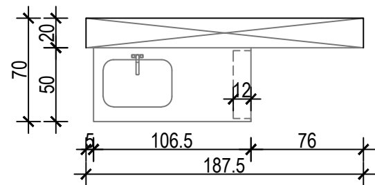
ELEMENT - TLOCRT
