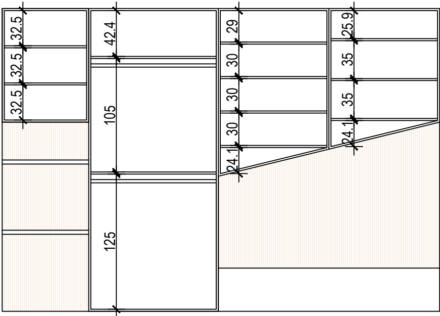
ORMAR - KORPUS
