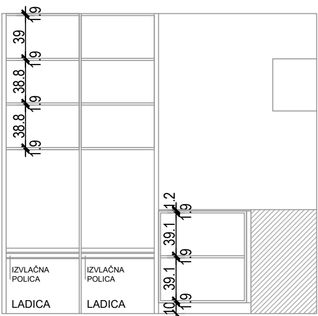
ELEMENT - KORPUS
