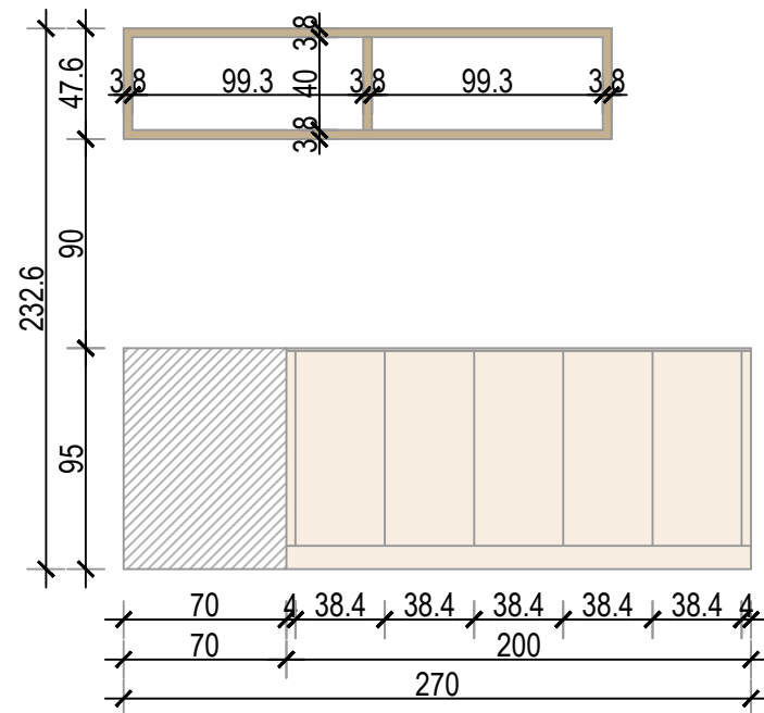
ELEMENT - POGLED
