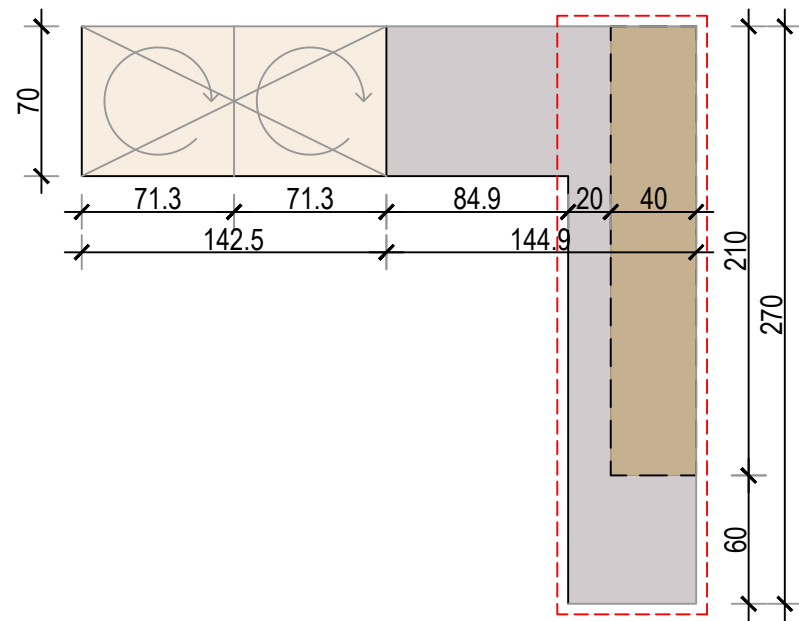
ELEMENT - TLOCRT
