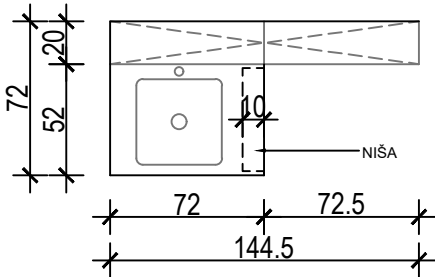
ORMAR - TLOCRT
