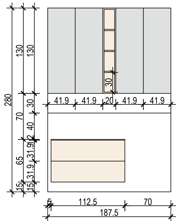
ELEMENT - TLOCRT
