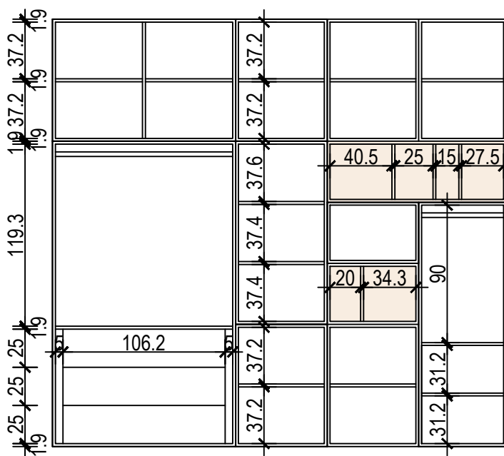
ORMAR - KORPUS
