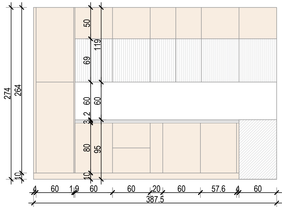
KUHINJA - POGLED
